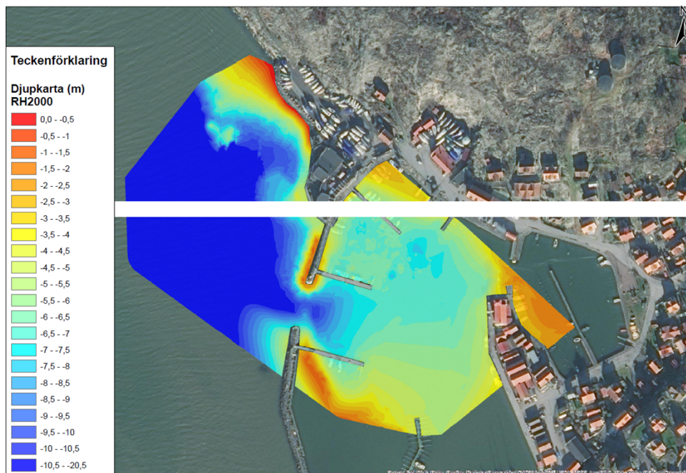
Bild 2. Djupkartering av Björkö fiskehamn
