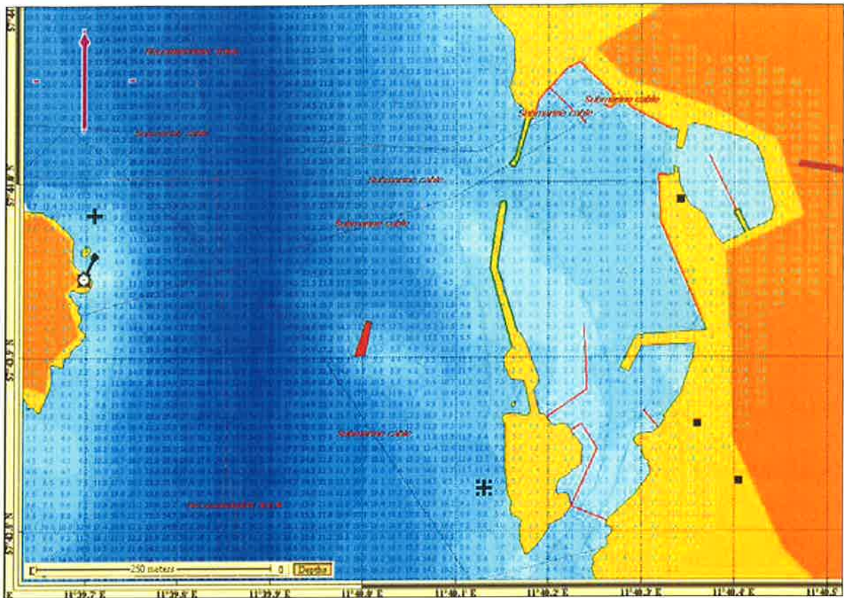
Djupförhållanden i meter. Djupangivelser nära och på land är extrapolerade och gäller ej.
