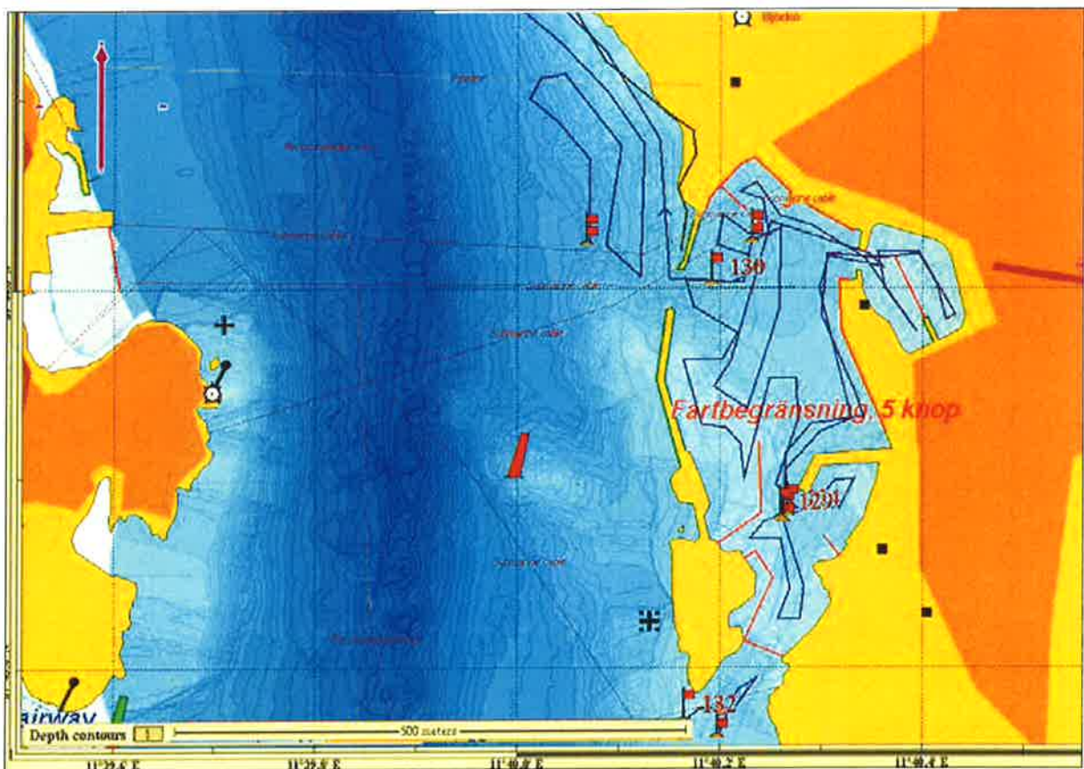
Avsökning med sidescan sonar 450 kHz.
